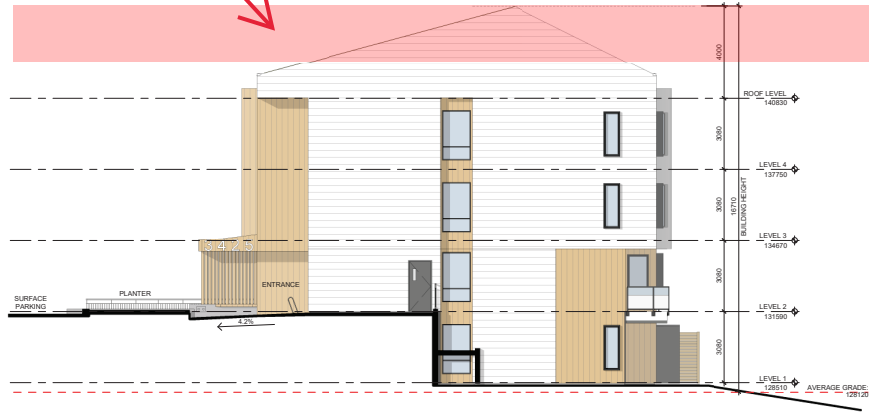
4 D07 ELEVATION - WEST D12 1:100
