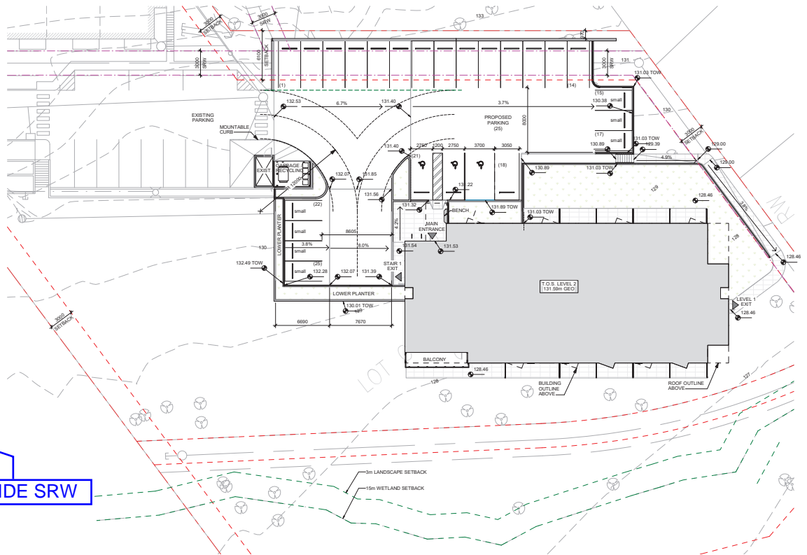
1 D06 SITE PLAN D06 1:200
