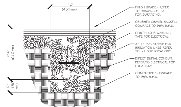
6 IRRIGATION SLEEVE L3 SCALE: 1-1/2" = 1' - 0"
