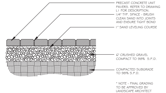
3 UNIT PAVING L3 SCALE: 1-1/2" = 1' - 0"
