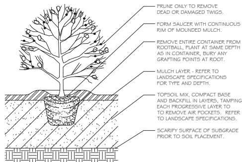
2 SHRUB PLANTING L3 SCALE: N.T.S.
