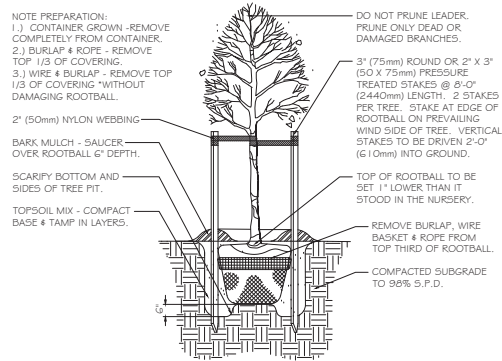
1 TREE PLANTING L3 SCALE: N.T.S.
