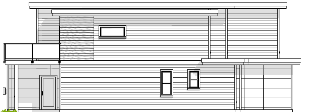
B RIGHT ELEVATION SCALE: 1/4" = 1'-0"
