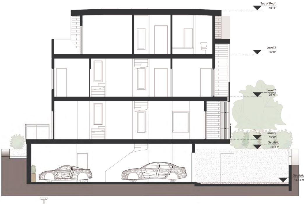
2 Section 2 Scale: 1/4" = 1'-0"
